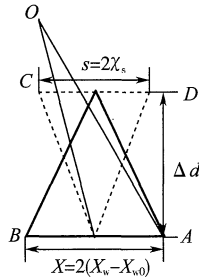
图 5 脱冰雪导线的运动范围示意图
