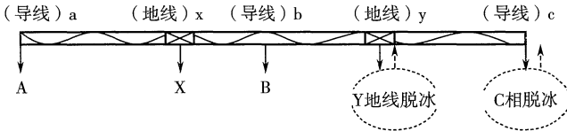
图 9 不均匀冰荷载组合示意图
