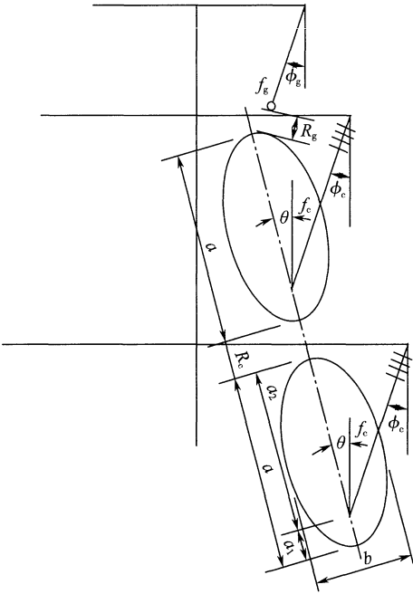
图 6 导线舞动时的电气间隙
